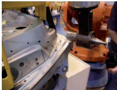
Rollhemming of a door
